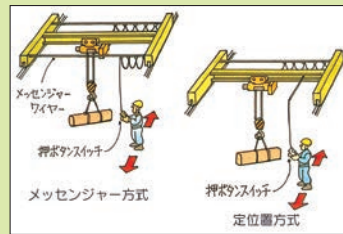
図3【床上操作式クレーン】
