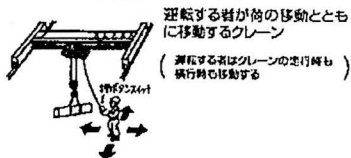
図3[床上操作式クレーン]
